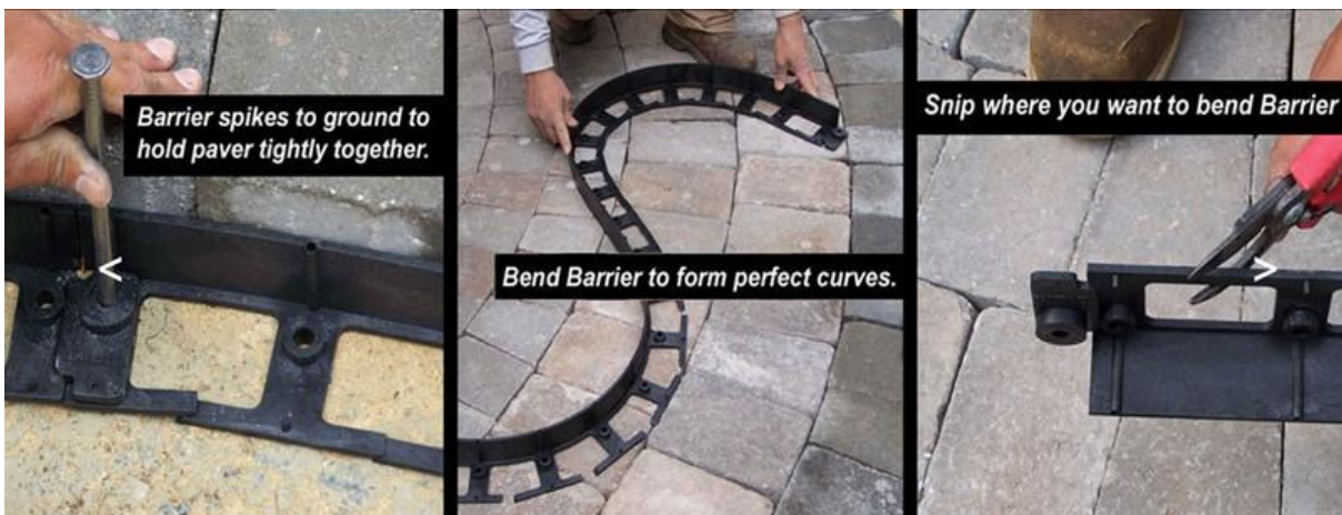
写真1 プラスチック製の端部拘束材(その1)
