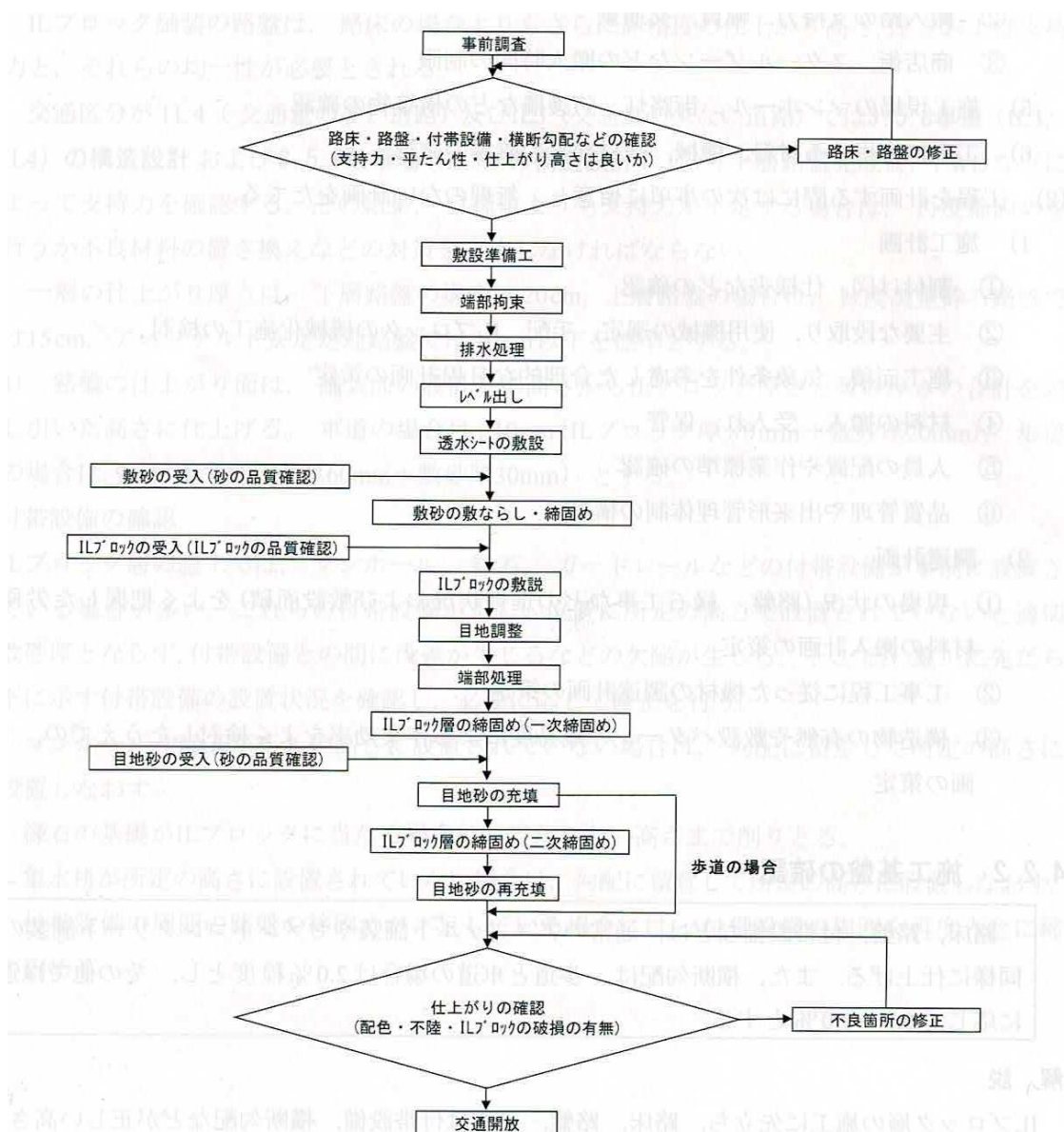
図1 IL ブロック層の施工フロー
